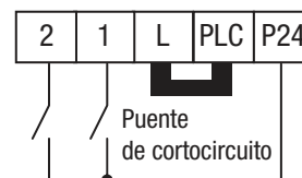
Lógica positiva
