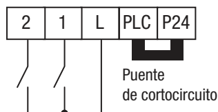
Lógica negativa
