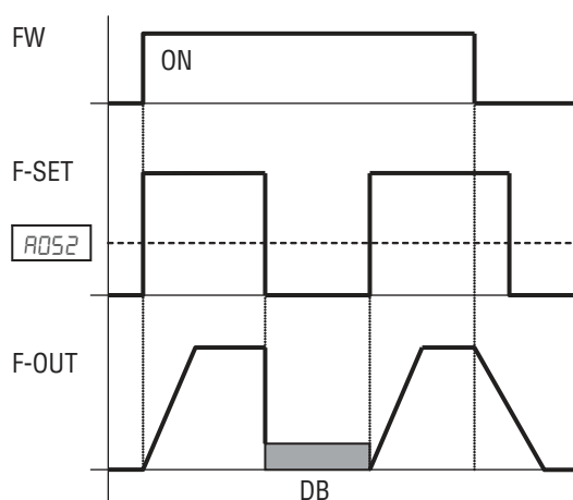
Ejemplo 1: cambio de paso en F-SET
